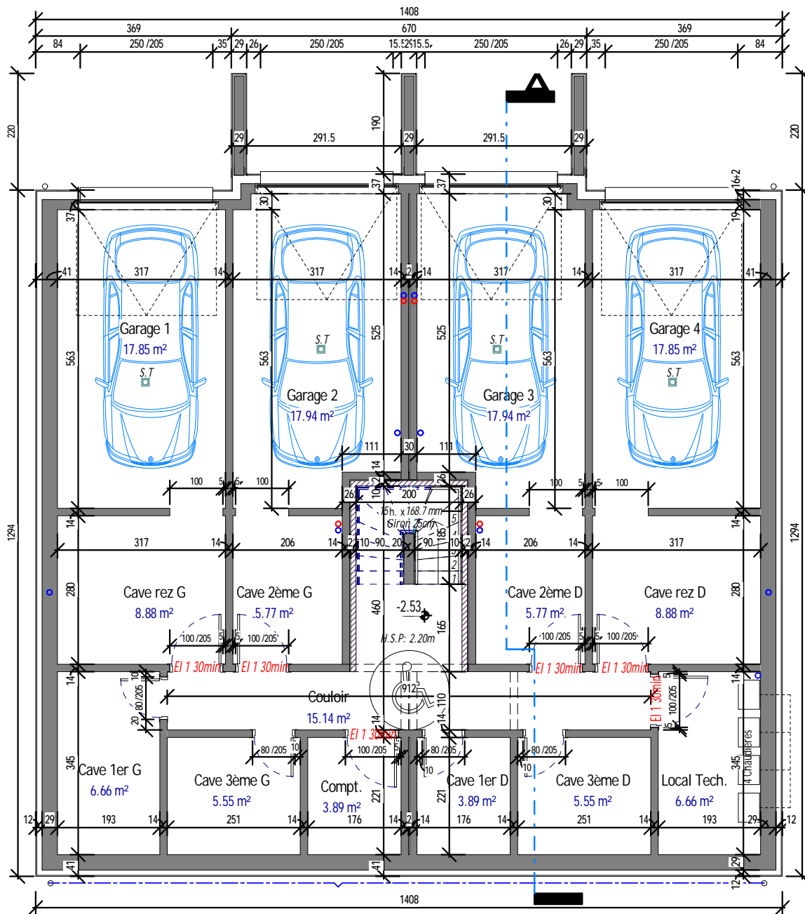
1 * -01 Sous-sol - Ech : 1 : 100
