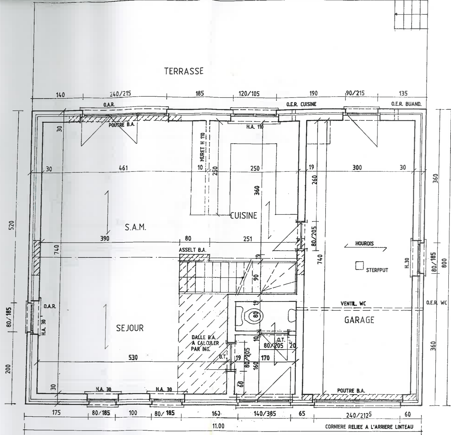
PLAN DESCRIPTIF COMPLET DU SYSTEME DE VENTIL. MANUELLE
